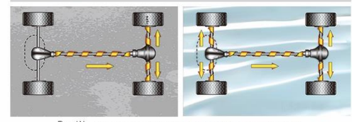
BorgWarner з електричним керуванням та повним приводом
